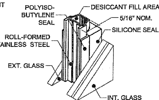
103 XL EDGE ™ SPACER
