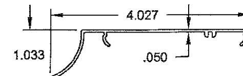
④ #8008 6063-T6 DRIP CAP
