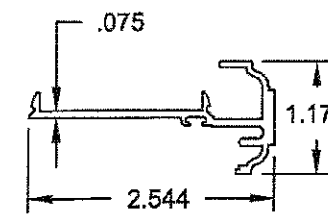
㉔ #8015 6063-T6 ASTRAGAL
