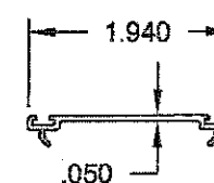
㉓ #8017 6063-T5 TOP SWEEP
