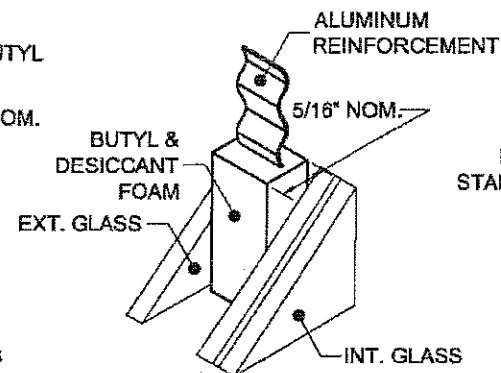
102 DURASEAL ® SPACER
