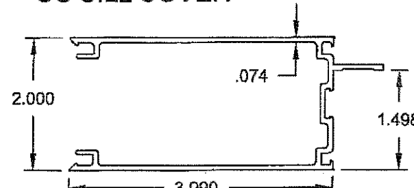
⑳ #8012 6063-T6 STILE
