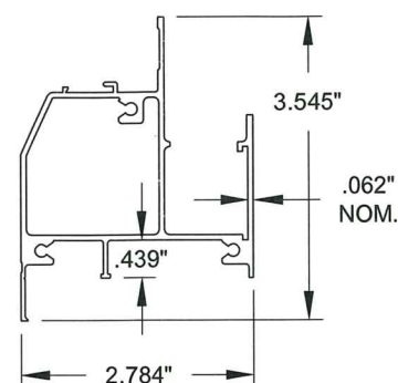
1 FRAME HEAD, SILL & JAMB #7005, 6063-T6
