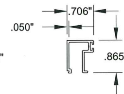
35 BEAD B #7036, 6063-T6
