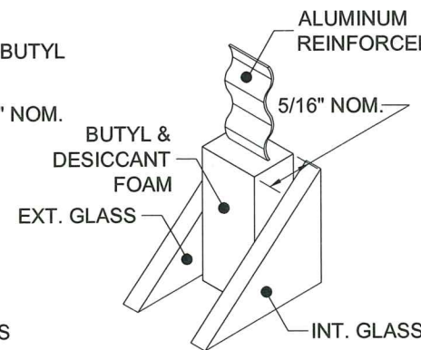
77 DURASEAL ® SPACER
