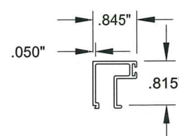
34 BEAD A #7037, 6063-T6
